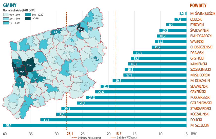
Wykres 2. Zainstalowana moc mikroinstalacji OZE na terenie województwa zachodniopomorskiego, stan na 31 grudnia 2023 roku (w MW)
